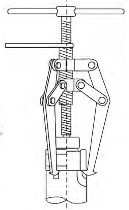
Извлечение внутреннего кольца с помощью инструментов для демонтажа
