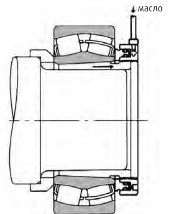
Извлечение при помощи гидравлической гайки
