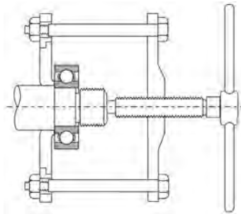
Извлечение внутреннего кольца с помощью инструментов для демонтажа
