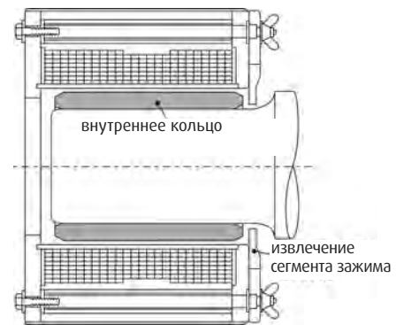
Извлечение внутреннего кольца при помощи индукционного нагревателя
